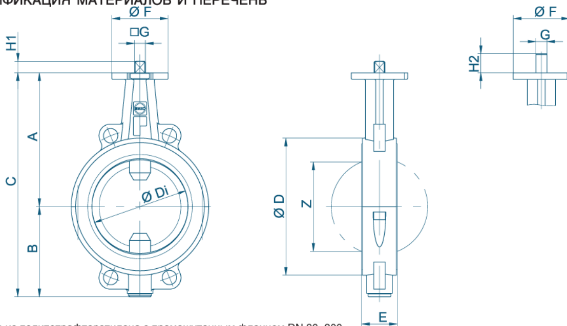
Заслонка из политетрафторэтилена с промежуточным фланцем DN 80–200
