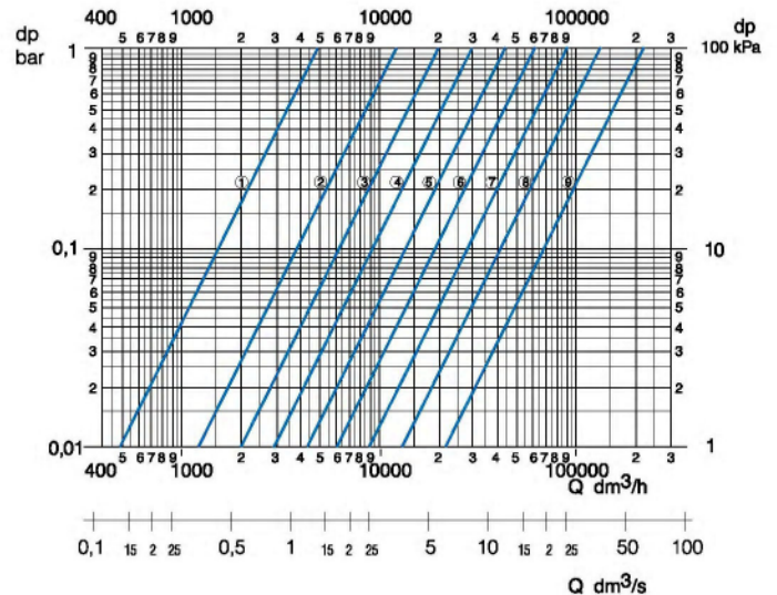
DN80
