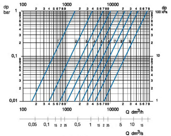
DN80
