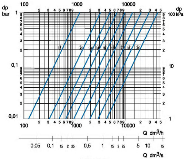
DN65
