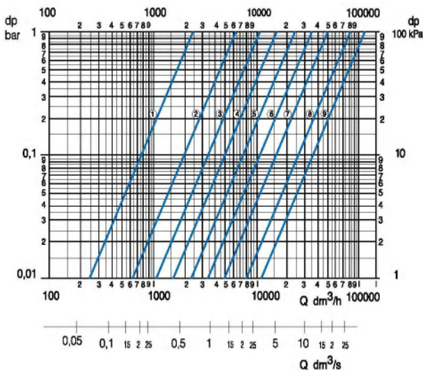
DN65
